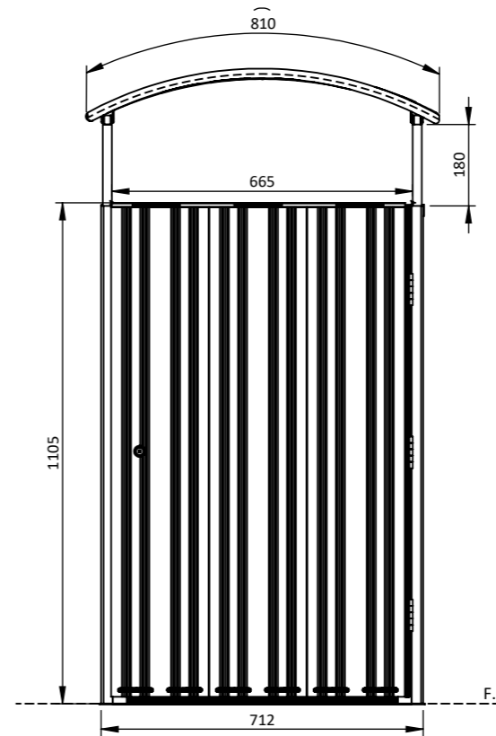
SIDE ELEVATION 1:15
